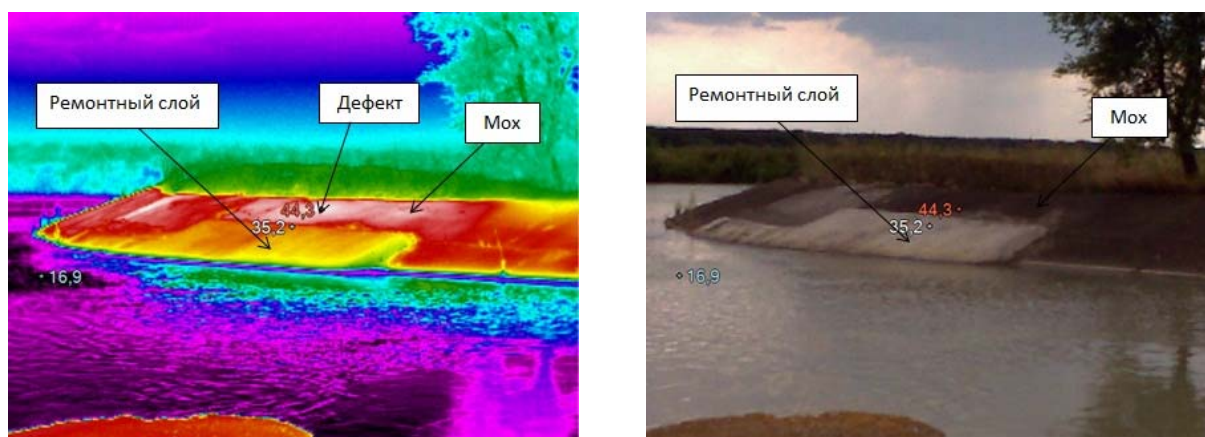
Рисунок 7. Обозначена зона дефекта, где было обнаружено отслоение. Ремонтный слой на термограмме может вызвать иллюзию дефекта, но на видимом режиме отчетливо видно, что это не дефект. Ещё одна аномалия, по температурному контрасту похожая на дефект, оказалось участком плиты, обросшим мхом
