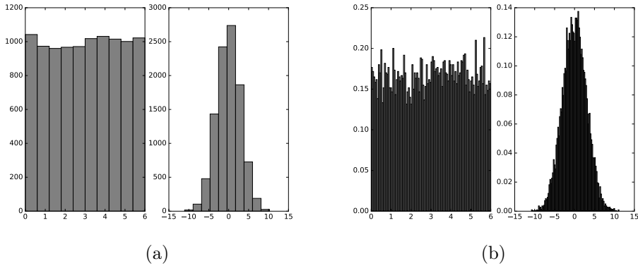
Рис. 5.6. Пример построения гистограмм: (a) — использованы значения параметров по умолчанию, в результате на обоих графиках наблюдаем по 10 бинов, а по вертикали отложено число попаданий в каждый из них; (b) — число бинов выставлено вручную и равно 100, по вертикали отложены значения плотности вероятности.
