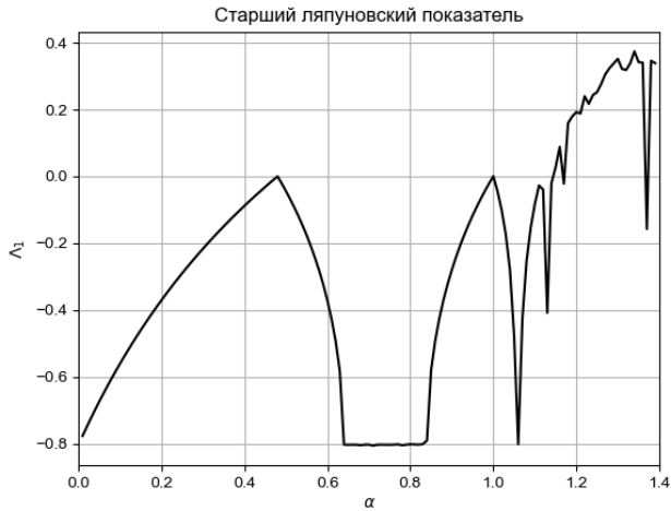
Рис. 12.18. Зависимость значения старшего ляпуновского показателя \Lambda_1 от параметра \alpha для отображения Эно.
