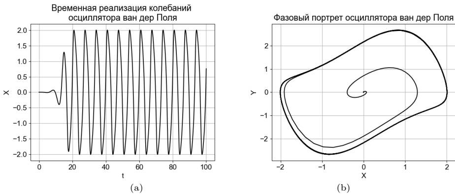
Рис. 12.8. Временная реализация колебаний (a) и фазовый портрет (b) осциллятора ван дер Поля.
