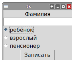
Рис. 11.7. Форма Tk, текстовое поле ttk.Entry , кнопка ttk.Button , метка ttk.Label , радиокнопка ttk.Radiobutton .
