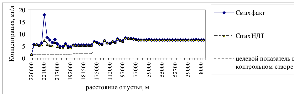
Рис. 4. Изменение максимальной концентрации БПКп по длине р. Луга при фактических концентрациях сброса и с учетом наилучших технологий
