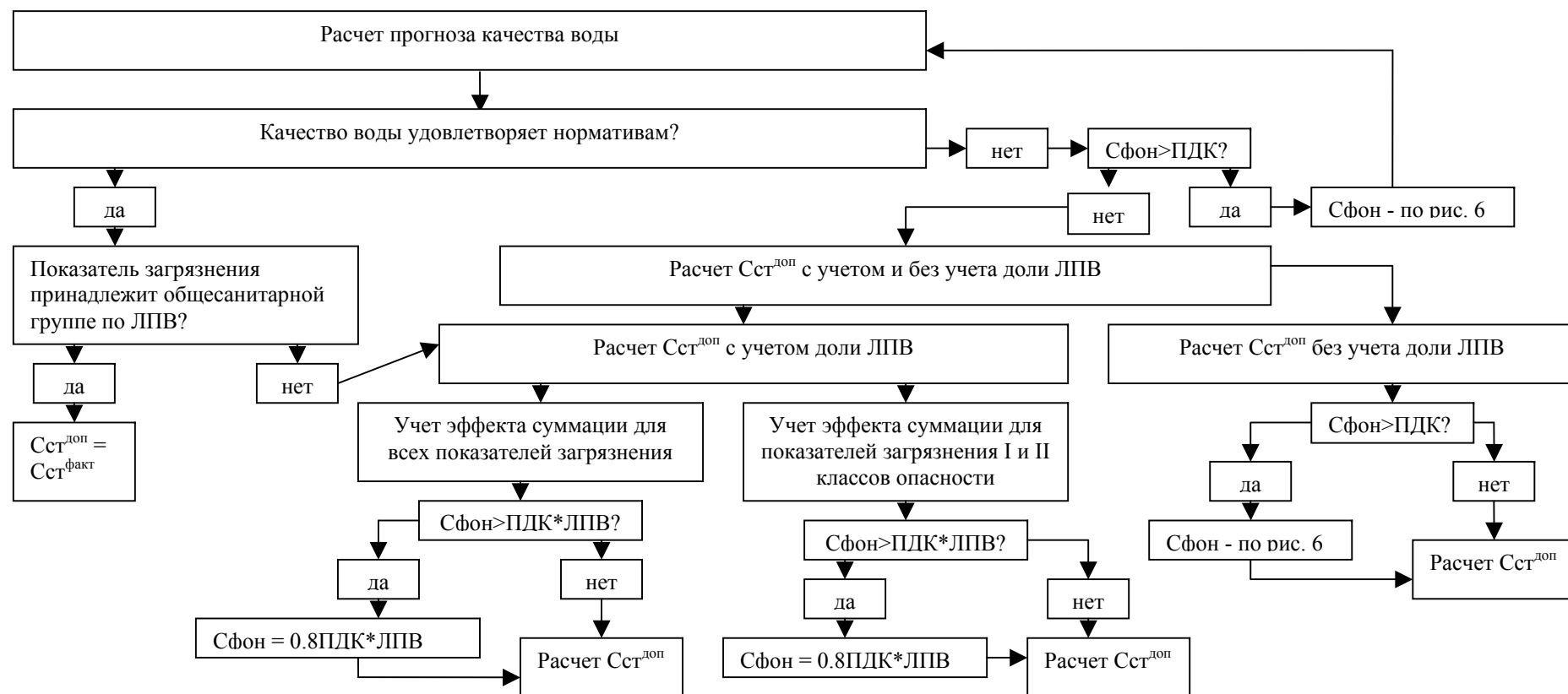
Рис. 7. Алгоритм прогноза качества воды и определения расчетных допустимых параметров сброса
