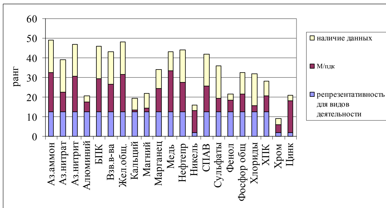
Рис. 9 Выбор основных показателей загрязнения р. Суйда
